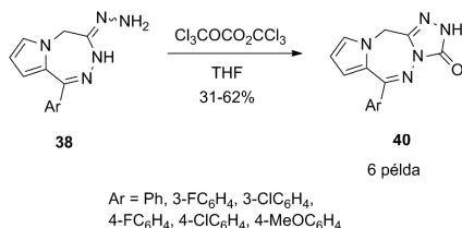
13. Ábra. Pirrolotriazolotriazepinon-származékok (40) előállítása.
