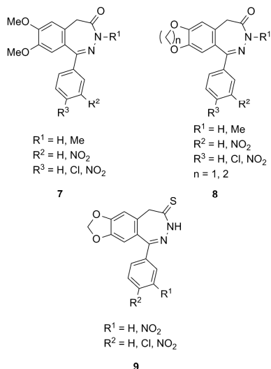
3. Ábra. 2,3-Benzodiazepin-4-on és tioanalóg vegyületek.
