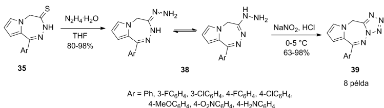
12. Ábra. Tetrazolopirrolotriazepinek (39) előállítása.
