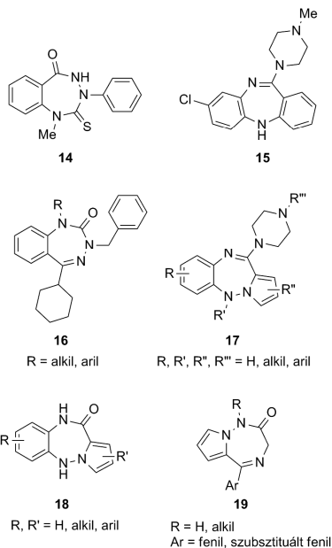
5. Ábra. Néhány jelentős triazepinszármazék.
