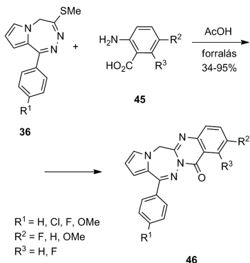
16. Ábra. Az előállított 46 kondenzált tetraciklusos.
