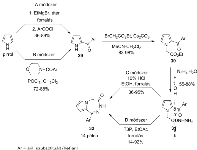
9. Ábra. 1-Aril-pirrolotriazepinon-származékok (32) előállítása.
