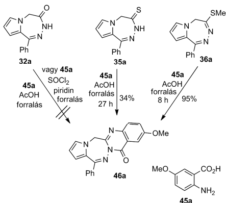
15. Ábra. Kísérletek a 46a vegyület előállítására.
