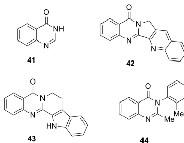
14. Ábra. Biológiailag hatékony kinazolinonszármazékok.
