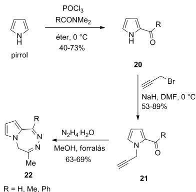
6. Ábra. A 22 pirrolotriazepinek szintézise.
