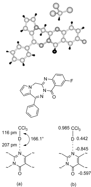
17. Ábra. A 46b vegyület szerkezete, (a) mért geometriai adatok, (b) számított töltéseloszlás.
