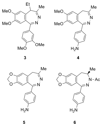
2. Ábra. Gyógyszerkémiailag szempontból jelentős 2,3-benzodiazepin-származékok.
