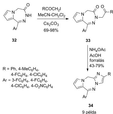
10. Ábra. Imidazolopirrolotriazepinek (34) előállítása.
