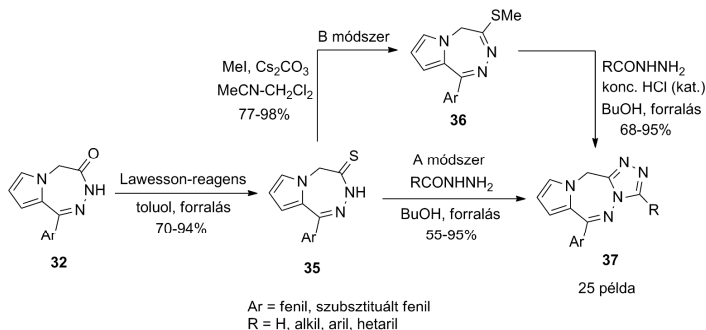
11. Ábra. Triazolopirrolotriazepinek (37) előállítása.
