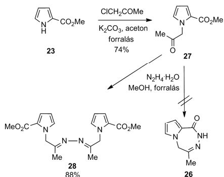
8. Ábra. Metil 1-(2-oxopropil)-1H-pirrol-2-karboxilát (27) reakciója hidrazin-hidráttal
