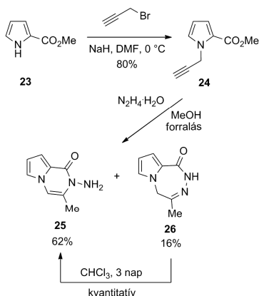
7. Ábra. A 25 pirrolpirazinon és a 26 pirrolotriazepin előállítása.
