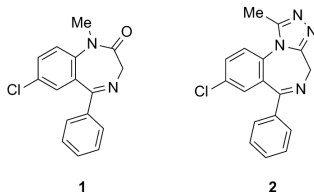
1. Ábra. A diazepam (1) és az alprazolam (2) szerkezete.
