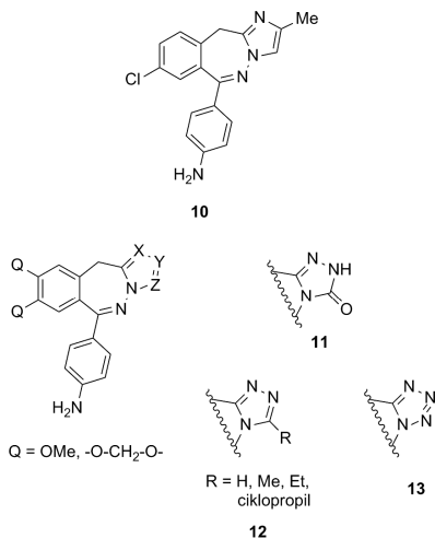
4. Ábra. Kondenzált triciklusos 2,3-benzodiazepinek.
