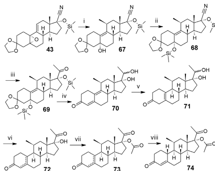
14. Ábra. A norgesztomet (74) szintézise.
