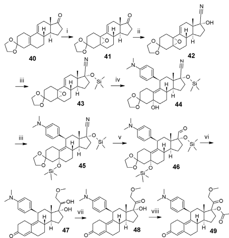
9. Ábra. Telaprisztion-acétát ( 49 ) előállítása.
