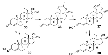
8. Ábra. Norgesztimét ( 37 ) és norelgesztromin ( 38 ) előállítása. i: Ac 2 O, HClO 4 ; ii: H 2 NOH; iii: LiOH; iv: H 2 NOH, HOAc
