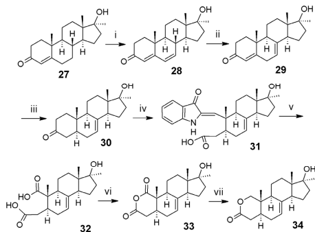
7. Ábra. \Delta^7 -oxandrolon (34) előállítása.
