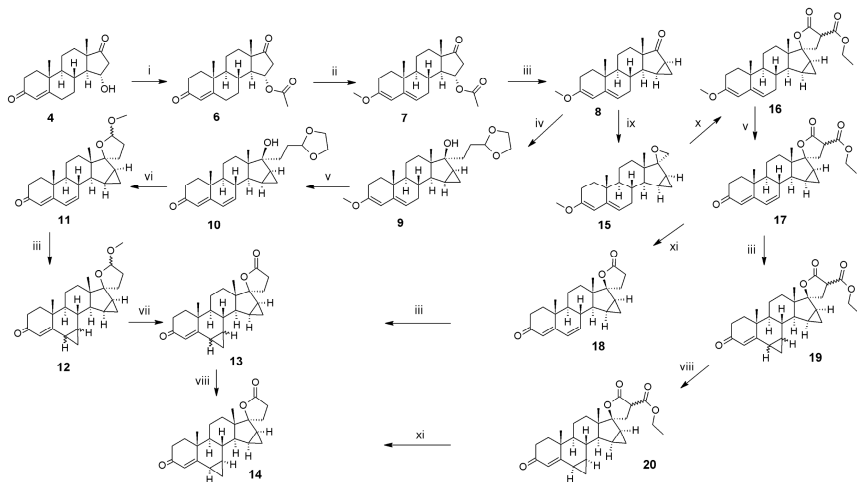
5. Ábra. A drospirenon (14) előállítása.
