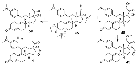
10. Ábra. Uliprisztál-acétát ( 1 ) és telaprisztion-acétát ( 49 ) előállítása közös intermediérből.
