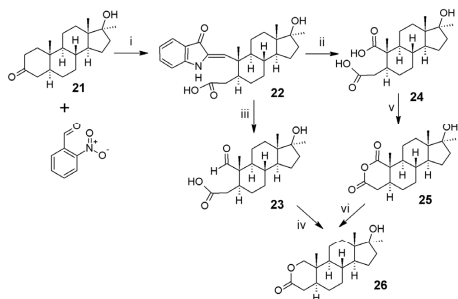
6. Ábra. Oxandrolon (26) előállítása.
