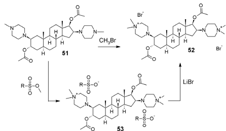
11. Ábra. A pipekuronium-bromid (52) szintézis zárólépése.
