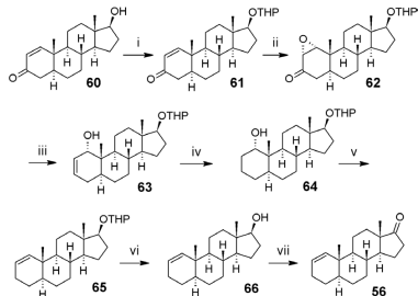
13. Ábra. Az 56 eliminációs melléktermék szintézise.
