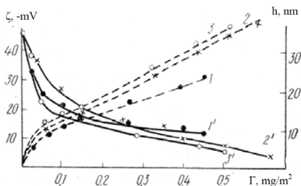
2. Ábra. 30 µm x 50 µm méretű grafitrészecskék elektrokinetikus potenciálja (1', 2', 3') és az ebből számított polimerreteg vastagsága (1, 2, 3) a polietilén-oxid, M=3 , 5 \cdot 10^5 (1, 1) M=10^6 (2, 2') és M=3 \cdot 10^6 (3, 3') adszorpciójának függvényében gyenge elektromos térben (6 V/cm), 10^{-4} M KCl oldat, szuszpenzió koncentráció 0,1 %.
