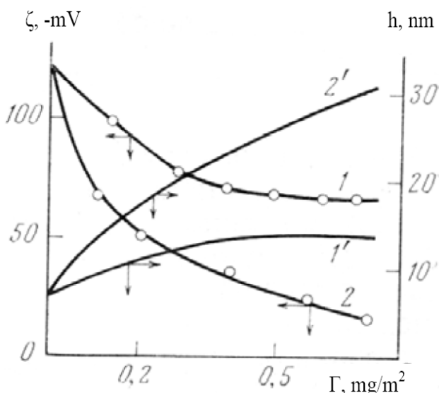
1. Ábra. 30 µm átmérőjű polisztirol részecskék elektrokinetikus potenciálja (1, 2) és az ebből számított polimerreteg vastagsága (1', 2') az adszorbeált polietilén-glikol, M=6 \cdot 10^3 (1, 1') és polietilén-oxid, M=3 \cdot 10^6 (2, 2') mennyiségének függvényében gyenge elektromos térben (6 V/cm), 10^{-4} M KCl oldatban, a szuszpenzió koncentrációja 0,06%.
