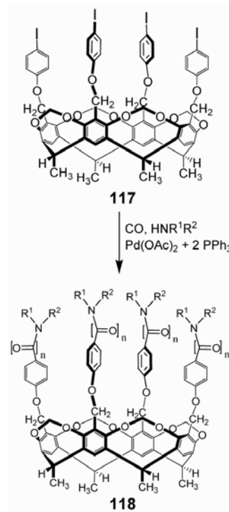
29. Ábra. Tetrajód-kavítand származék aminokarbonilezése.
