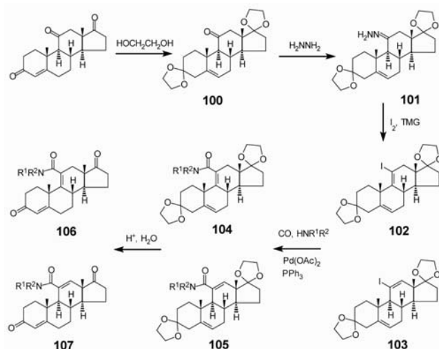
26. Ábra. 11-Karboxamido-3,17-dion származékok kialakítása adrenoszteron kiindulási anyag alkalmazásával.
