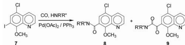
4. Ábra. 8-Metoxi-5-klór-7-jód-kinolin aminokarbonilezése.
