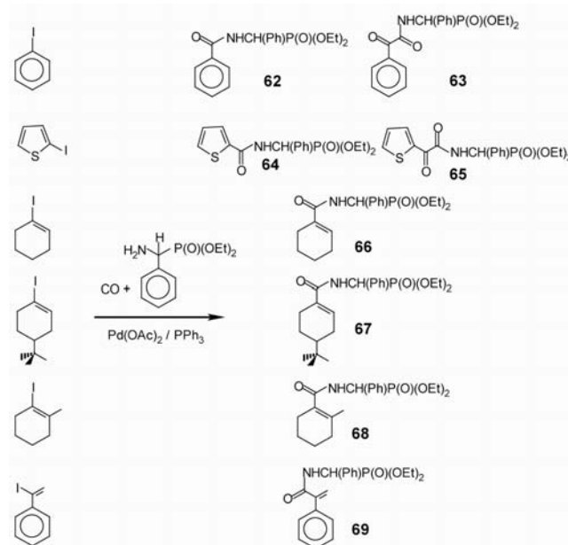
18. Ábra. Dietil- \alpha -amino-benzilfoszfónát mint N -nukleofil alkalmazása jód-aromás és jód-alkének aminokarbonilezési reakciójában.
