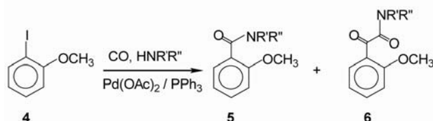
3. Ábra. 2-Jód-anizol aminokarbonilezése.
