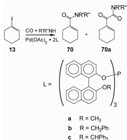
19. Ábra. 1-Jód-ciklohexén kettős karbonilezési reakciója foszfitek mint ligandumok jelenlétében.
