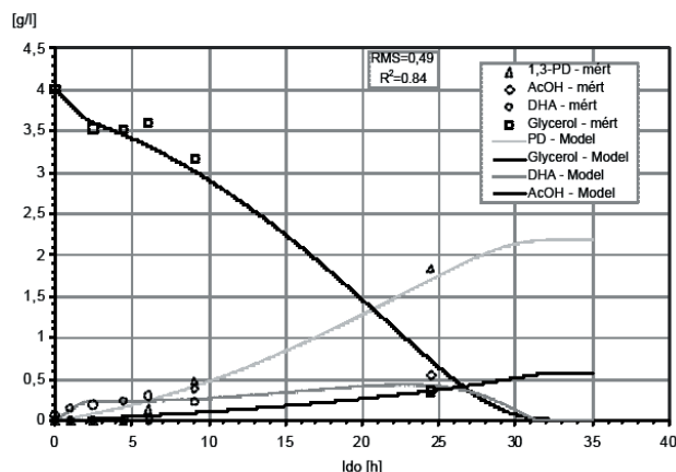
2. Ábra. Glicerinn biokonverzió Klebsiella eredetű enzimekkel: mért és illesztett koncentrációk ( Y_{1,3PD} =46%, Y_{DHA} =10%, Y_{AcOH} =15%, Konverzió: 88%).
