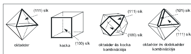
5. Ábra .Gyémánt kristályformák
